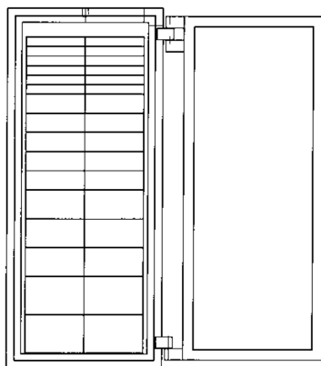
Wertschutzschrank Modellreihe 1901 mit 32 Mietfächern und versperrbarem Innenfach
